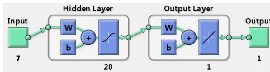
شکل ۴. شبکه عصبی اجرا شده توسط نرم افزار MATLAB
