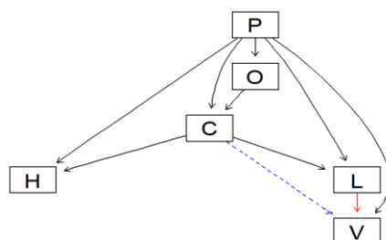
شکل ۶. مقایسه شبکه باور بیزی روزانه و هفتگی
