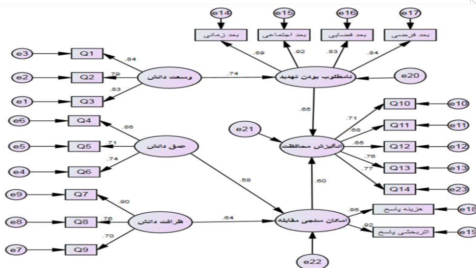
شکل ۲: مدل پژوهش با ضرایب استاندارد شده بار عاملی (ارزیابی مدل‌های اندازه‌گیری) پیش از بررسی فرضیه‌ها شاخص‌های برازش باید بررسی شوند:
