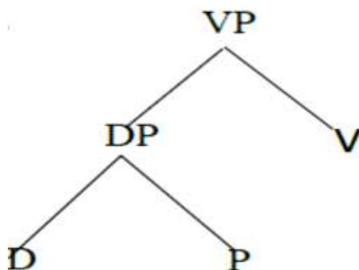
شکل ۱. حرکت هسته‌به‌هسته
