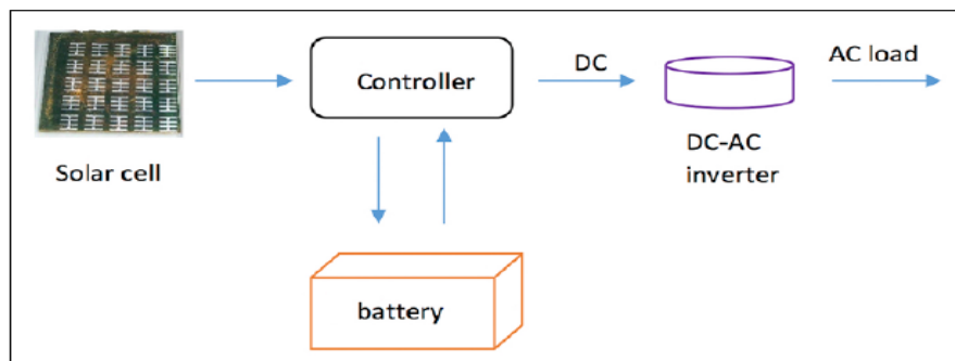
شکل ۱. تصویر برد سلول خورشیدی سامانه واحد انرژی تجدیدپذیر.
