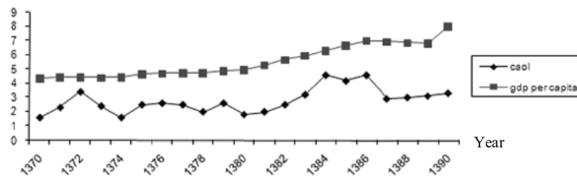
شکل ۱. مصرف زغال سنگ و تولید ناخالص داخلی سرانه (کشور ایران)
