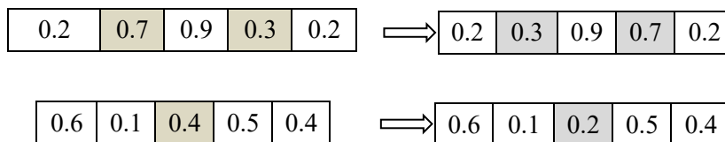
شکل ۴. عملگرهای جهش
