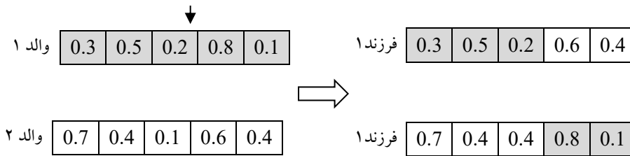
شکل ۳. عملگر تقاطع تک نقطه ای
