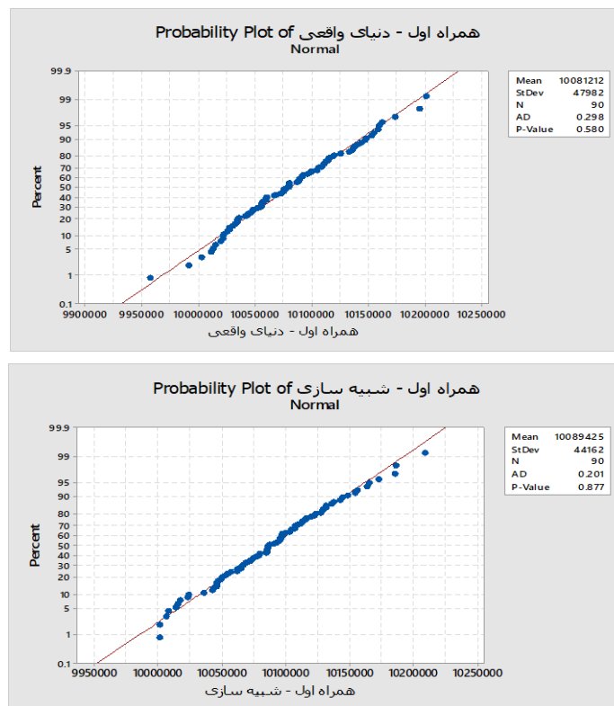
شکل ۱۱. آزمون نرمال بودن داده‌های شرکت همراه اول در دنیای واقعی و نرم‌افزار شبیه‌سازی
