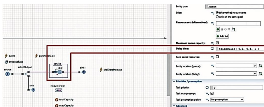
شکل ۵. استفاده از تابع توزیع مثلثی در نرم‌افزاری لاجیک
