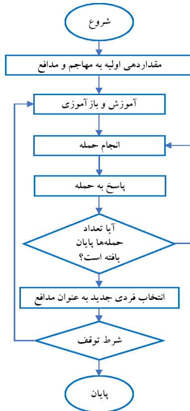
شکل ۸ فلوجارت SEO
