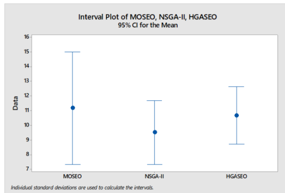
شکل ۲۰. نمودار فاصله‌های NPS (فاصله اطمینان ۹۵٪)
