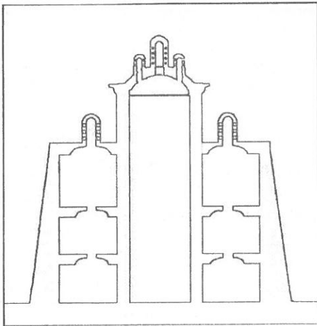
تصویر شماره ۲: نمایی از یک کبوترخانه سه طبقه دوجداره (میرزایی)
