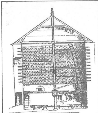
تصویر شماره ۱: اجزای کبوترخانه استوانه‌ای شکل در انگلستان (کوک، ۱۹۲۰)
