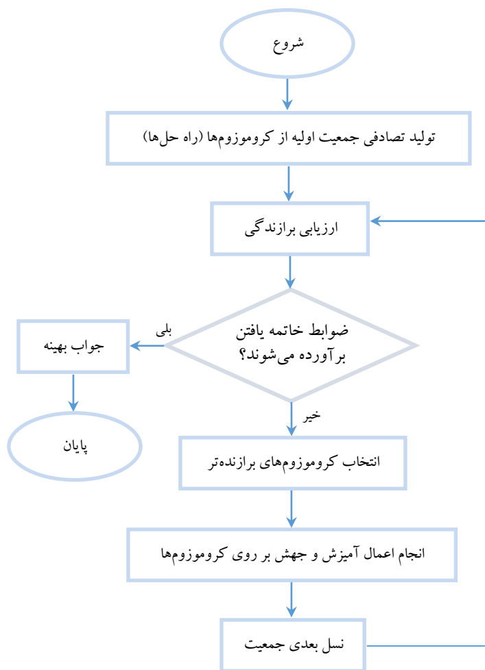
شکل ۴: فلوچارت الگوریتم ژنتیک استاندارد
