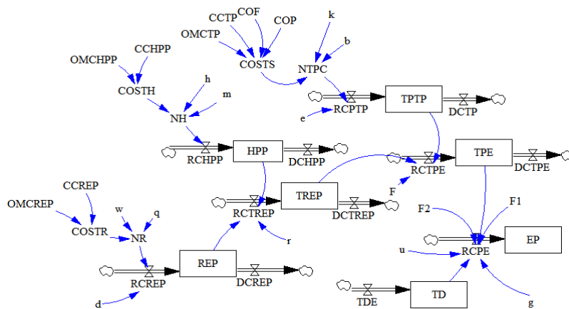
نمودار (۷): نمودار جریان مدل
